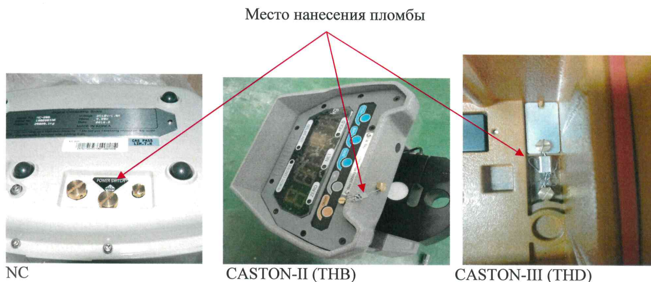
Рисунок 2 - Место пломбировки весов
