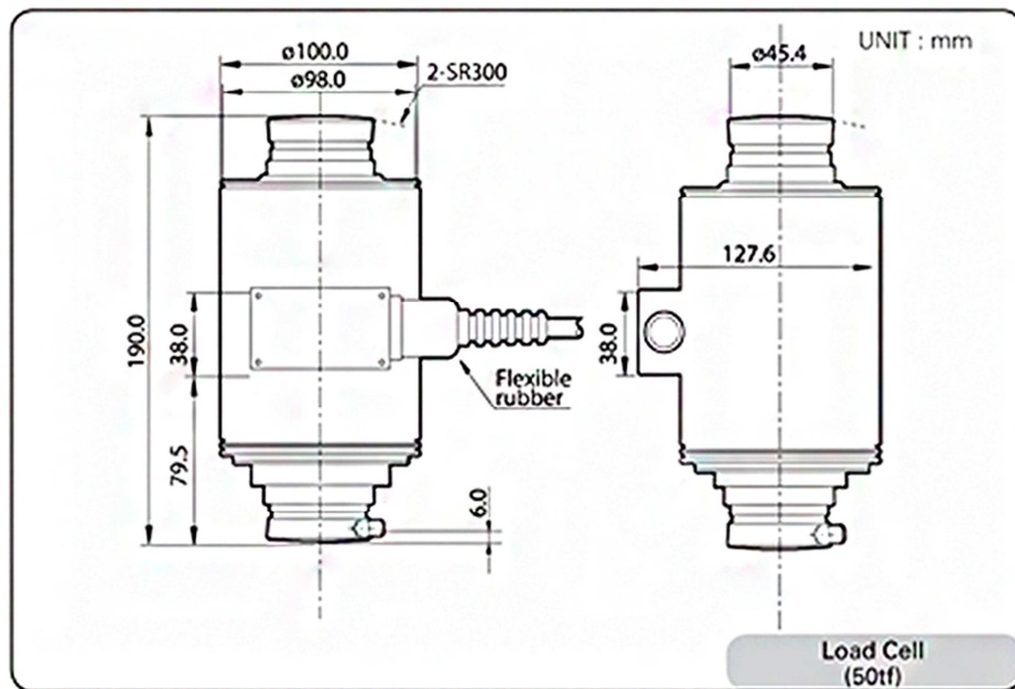
Размеры тензодатчика WBK TL (50tf) с аксессуарами WBK-LOW
