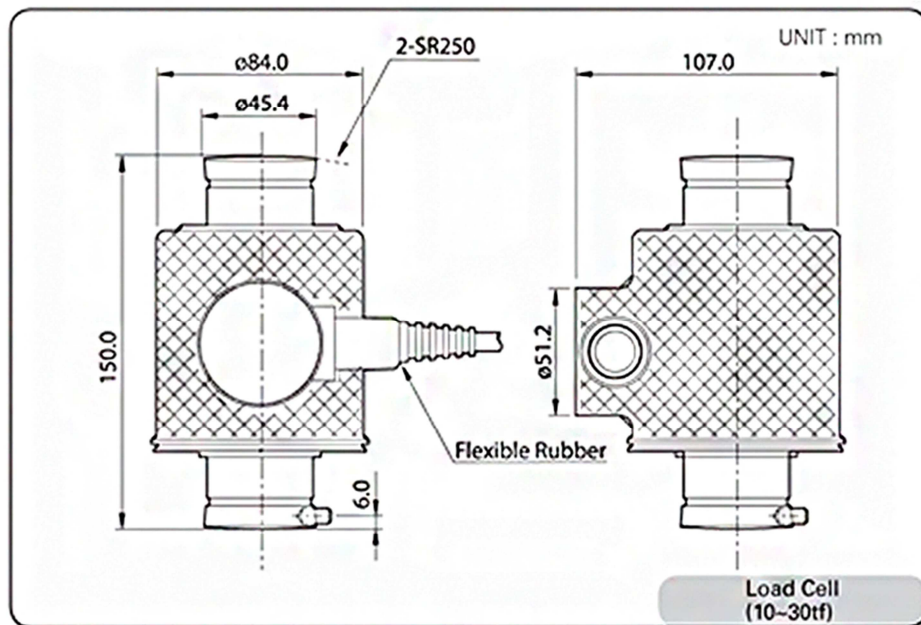
Размеры тензодатчика WBK TL (10-30tf) с аксессуарами WBK-LOW
